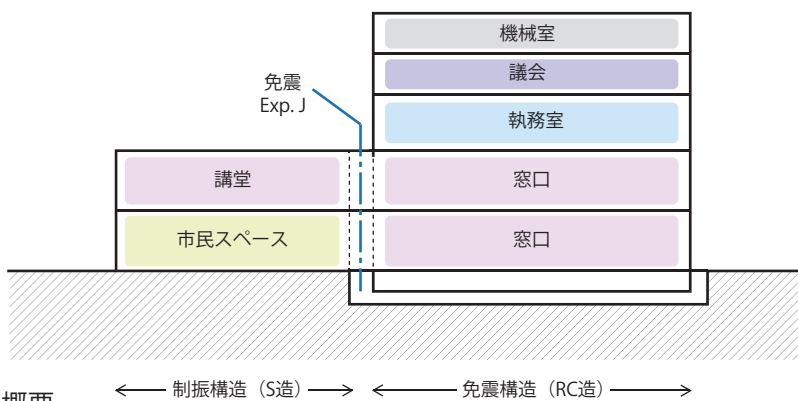
断面概要 ← 制振構造 (S造) → ← 免震構造 (RC造) →
